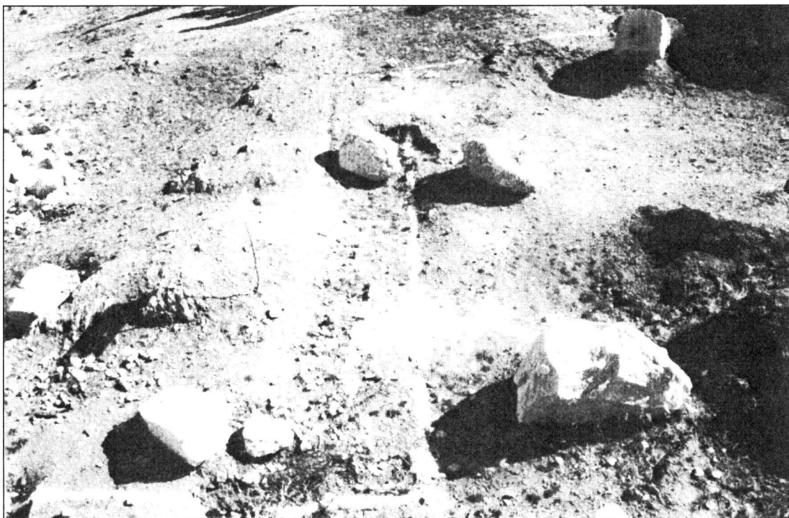
(تصویر - ۱۶): ته رنگ جاسازی بستر سنگ های نمای وجوه از میان رفته پلکان شمالی و تختگاه کوچک مهتابی شرقی بر صخره طبیعی، گنج ریزی شالوده طرح بازسازی گوشه شمال شرقی تختگاه.
