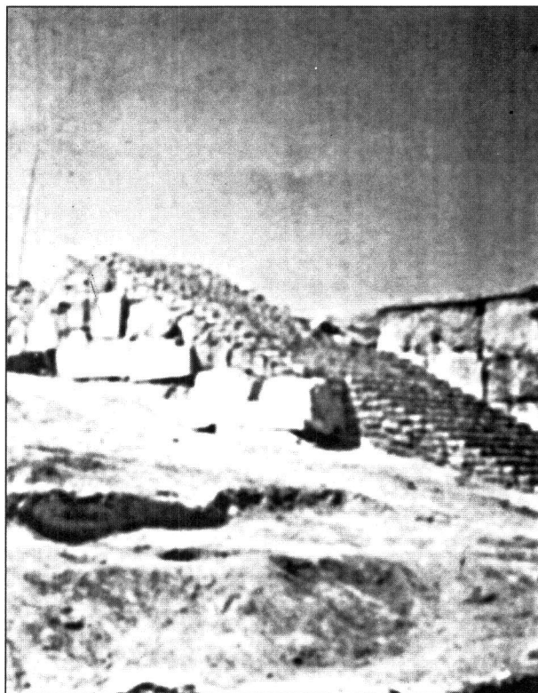
(تصویر - ۲۱. ب.): آجر فرش بالای سنگ‌های نمای مهتابی شرقی از شدت آسیب تابش آفتاب و یخبندان زمستان کنگاور می‌کاهد.
