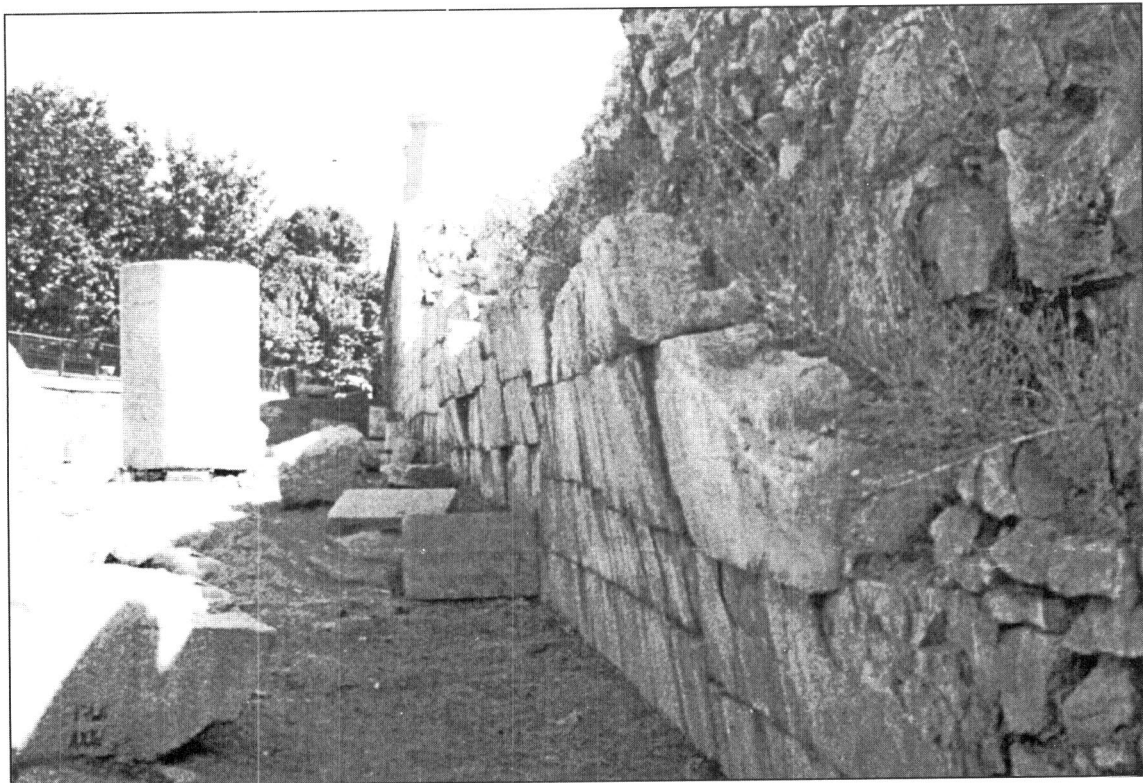
(تصویر-۶): آسیب‌های عمومی نمای جبهه غربی در راستای بخش بازسازی شده.
