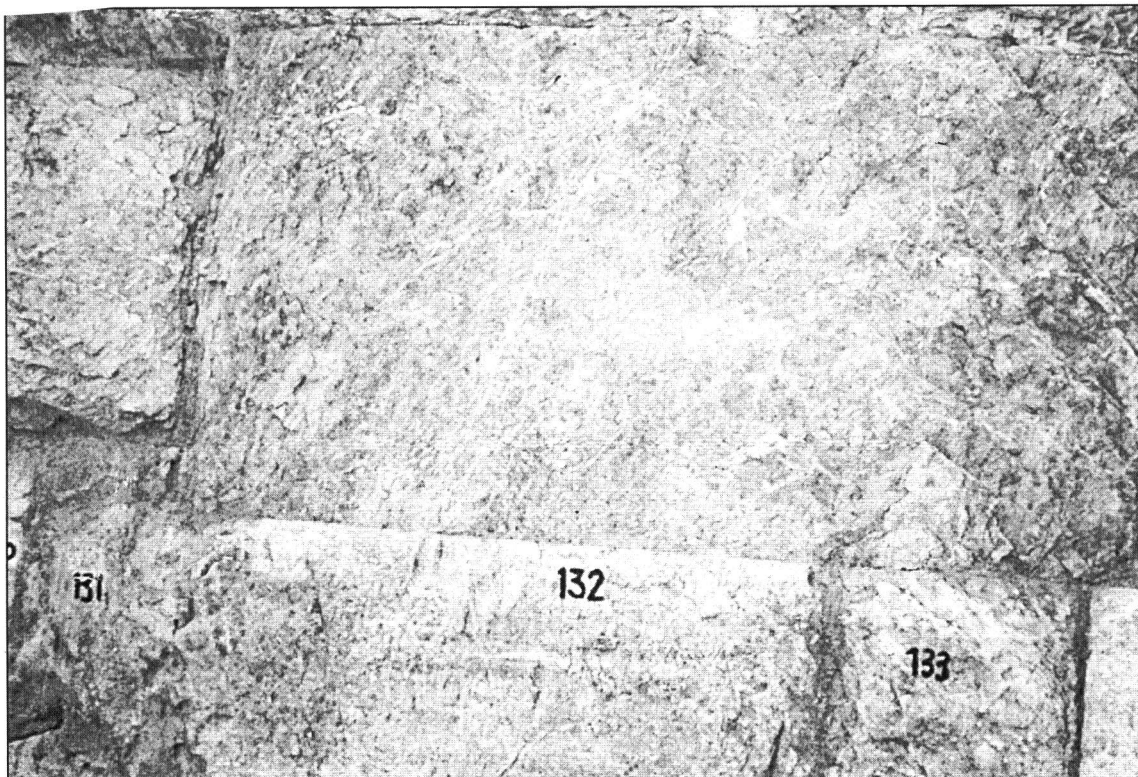
(تصویر-۸): درزبندی سنگ‌های نمای آسیب‌دیده و پیاده نشده در میان بخش بازسازی شده جبهه غربی معبد اناهیتا.
