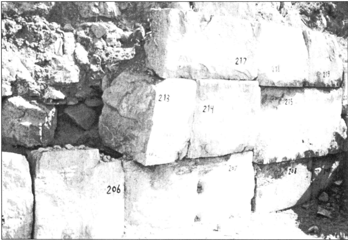
(تصویر-۷): آسیب‌های ناشی از آبشستگی ملاط سطوح زیرین مهتابی جبهه غربی وانحراف سنگ‌های تحتانی نما.
